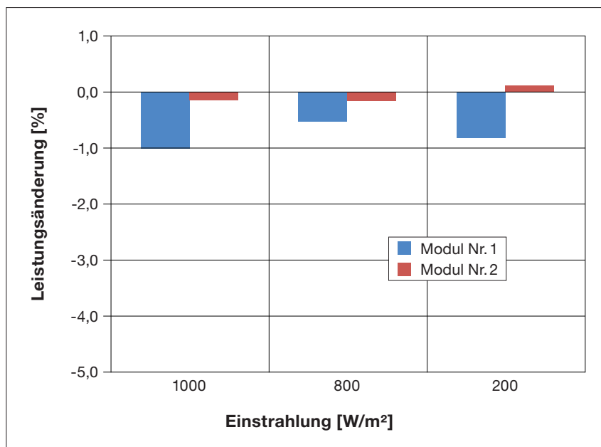
Bild 1: Leistungsänderung nach dem Klimatest unter Ammoniakatmosphäre
