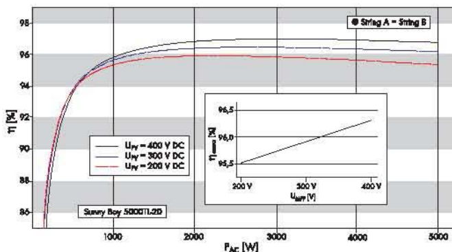
Wirkungsgradkurve
